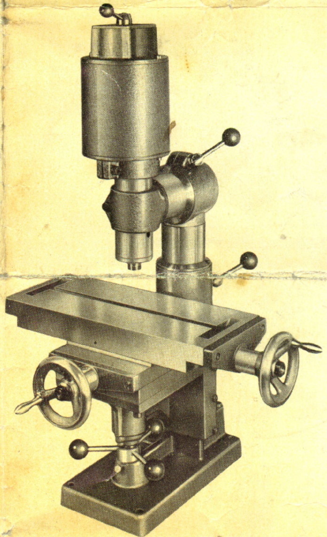
Vertikalfräsmaskin
